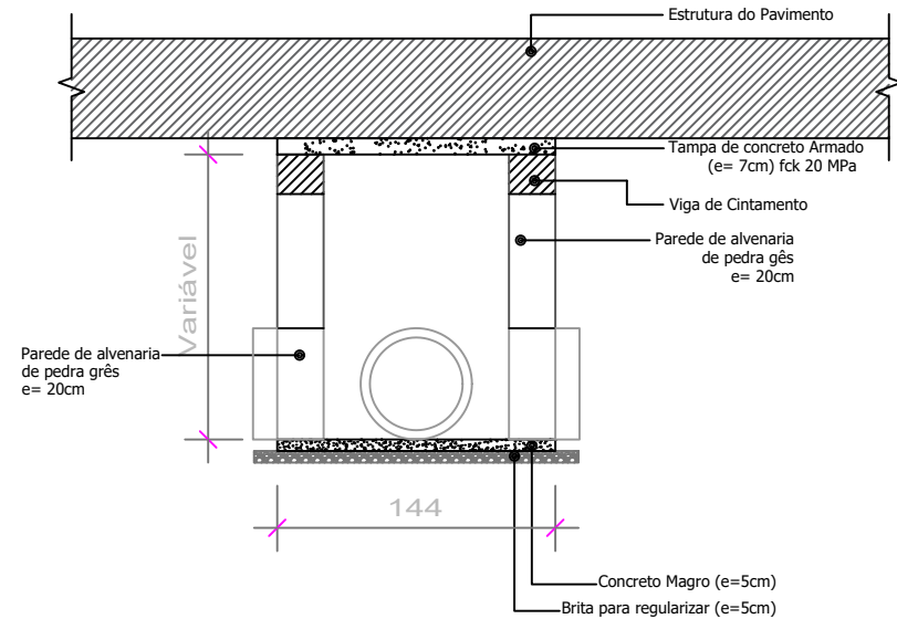
CORTE A-A' - CAIXA HIDRAULICA ENTERRADA (1,00 x 1,00m int.) Sem escala Obs.: A altura total da caixa coletora poderá variar conforme as características do terreno no local de sua execução, com altura até 1,50m.
