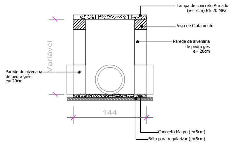
CORTE A-A' - POÇO DE VISITA (1,00 x 1,00m int.) Sem escala Obs.: A altura total da caixa coletora poderá variar conforme as características do terreno no local de sua execução, com altura até 1,50m.
