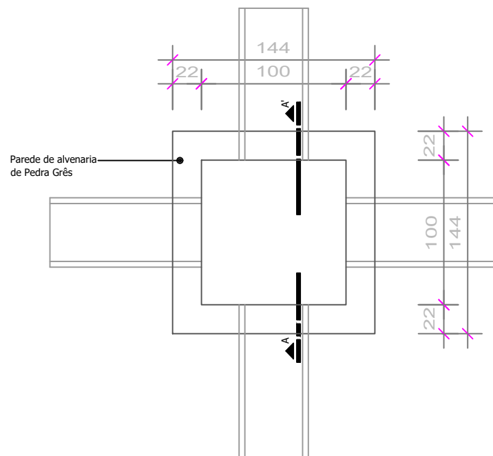
PLANTA BAIXA - CAIXA HIDRAULICA ENTERRADA (1,00 x 1,00m int.) Sem escala
