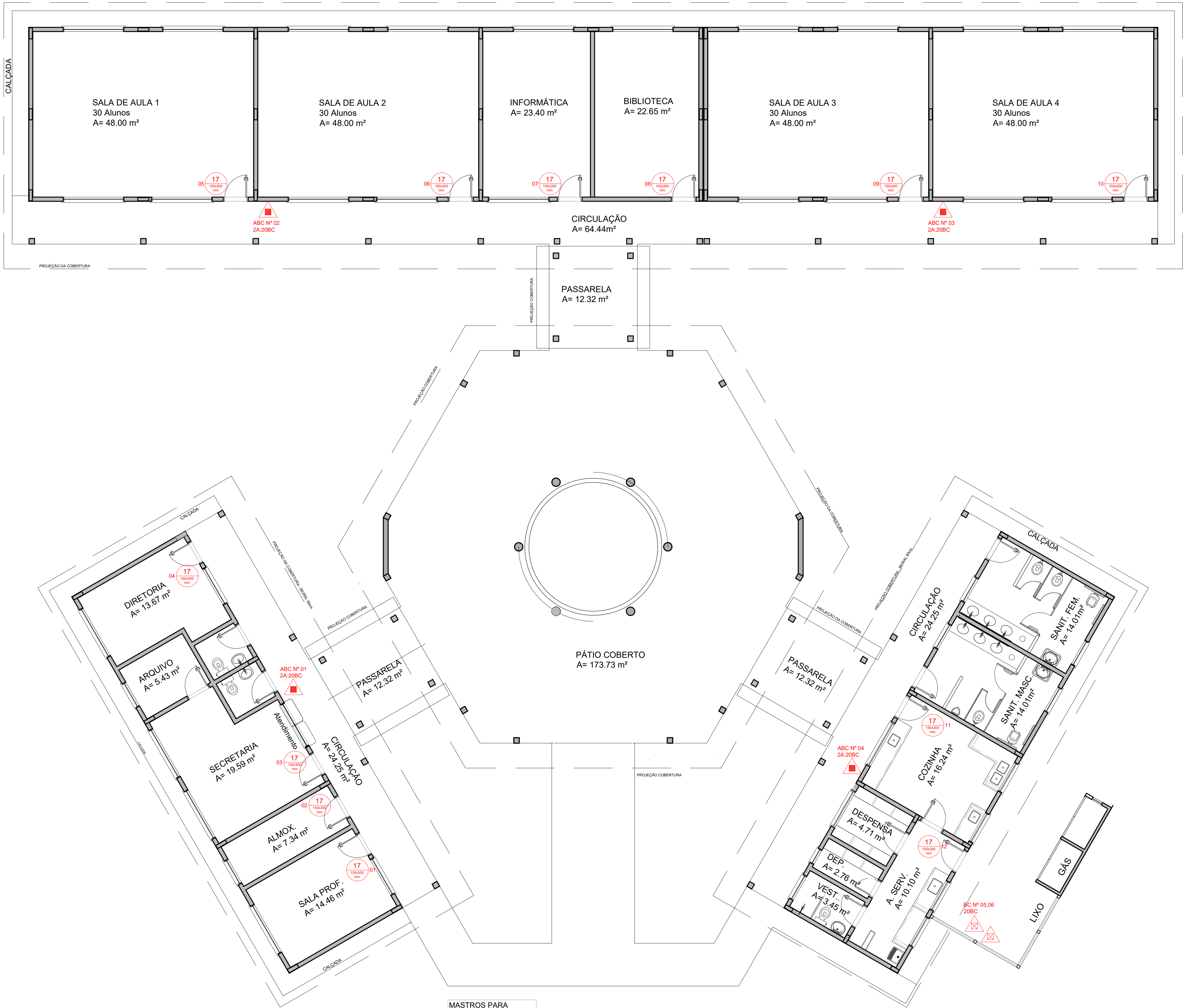
PLANTA BAIXA PAV. TÉRREO Esc 1:75
