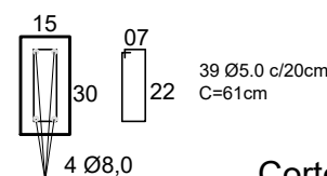
Corte Viga esc. 1/25
