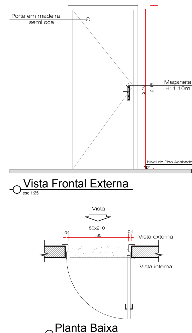
Planta Baixa esc 1:25
