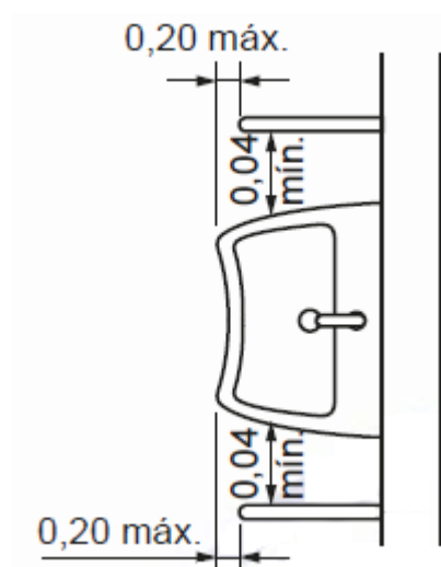
Figura 20 - Planta baixa instalação de barras laterais horizontais ao lavatório
