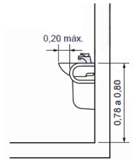
Figura 21 - Vista lateral de instalação de barras laterais horizontais ao lavatório
