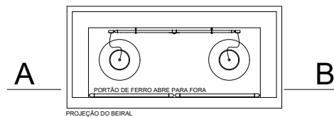
CENTRAL DE GÁS PLANTA BAIXA
