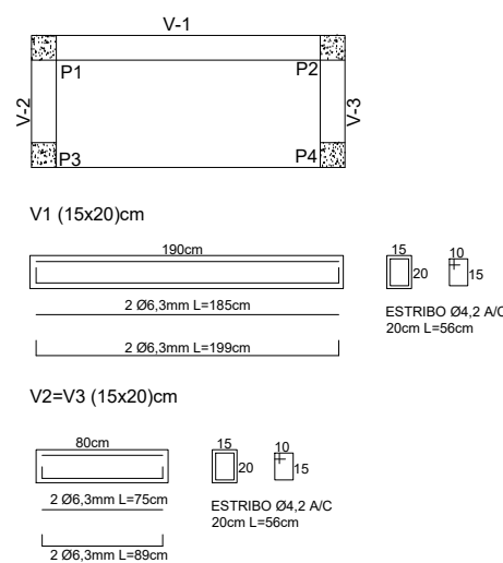
ESTRUTURAL: Vigas de amarração
