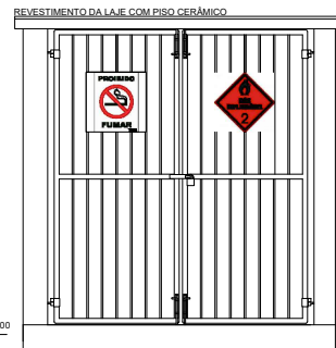
CENTRAL DE GÁS FACHADA LATERAL
