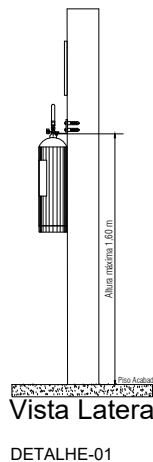
CENTRAL DE GÁS FACHADA LATERAL
