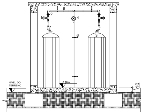
CENTRAL DE GÁS CORTE (AB)
