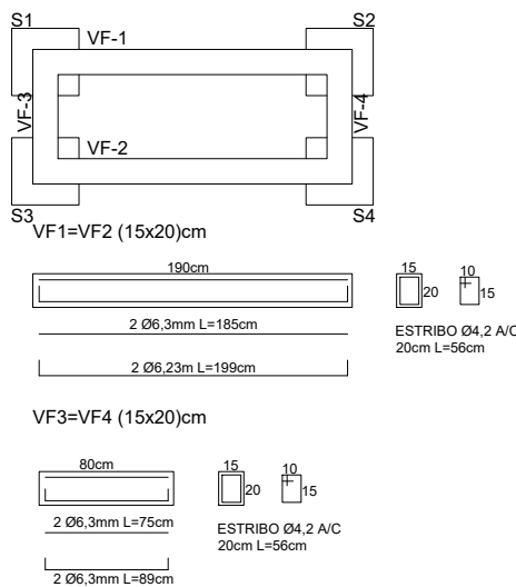
ESTRUTURAL: Vigas de fundação
